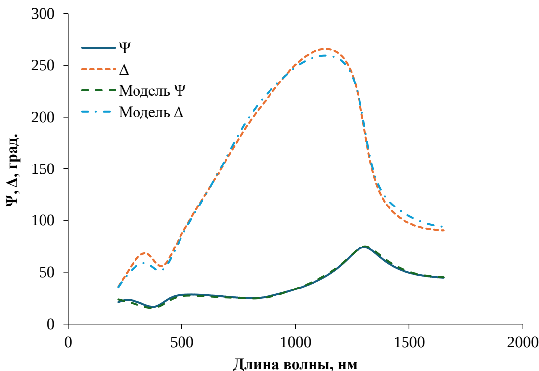
Рисунок 3.14 – Спектральные зависимости параметров \Psi и \Delta для экспериментальных данных и расчетной модели образца В 4 С-200
