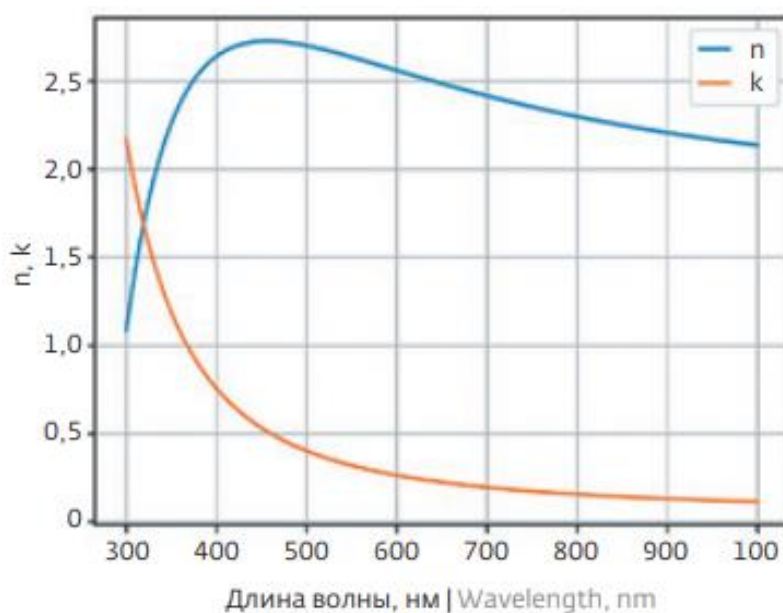
Рисунок 1.5 – Показатели преломления (n) и поглощения (k) пленки \text{W}_4\text{C} толщиной 850 нм
