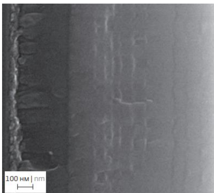
Рисунок 1.2 – Слоистая и столбчатая структура B_4C , полученная при температуре 200 °С и давлении Ar 0,187 Па
