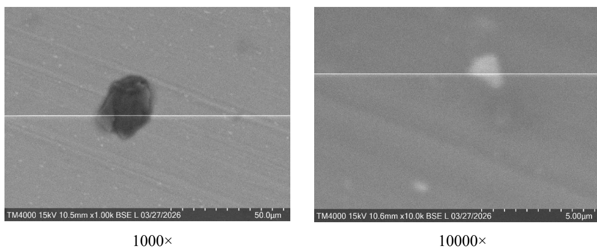
Рисунок 3.8 – СЭМ-изображения первого участка образца В 4 С-400 при приближении 1000× и 10000× в режиме BSE
