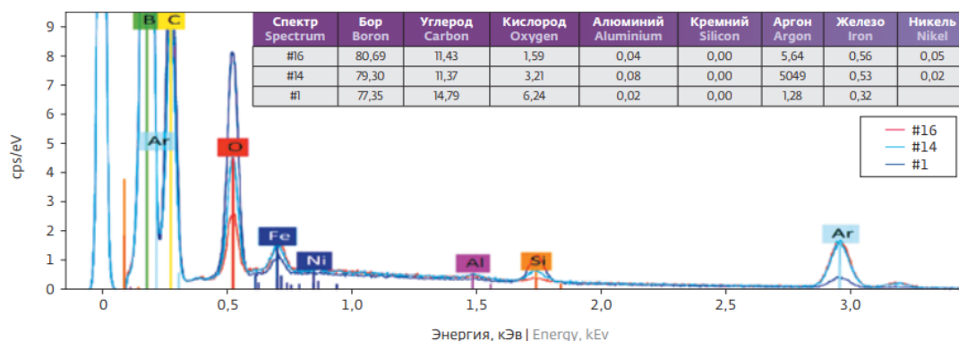
Рисунок 1.4 – Энергодисперсионные рентгеновские спектры пленок В 4 С, полученных без ионного ассистирования (образец № 1) и с применением ионного ассистирования (образцы № 14 и № 16)
