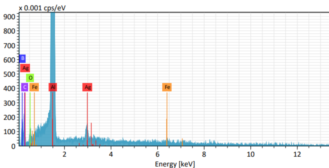
Рисунок 3.7 – ЭДС-спектр образца В 4 С-200
