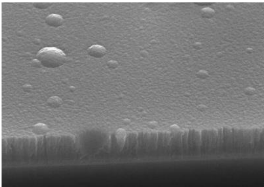
Рисунок 1.1 – Столбчатая структура В 4 С, полученная при 400 °С и давлении Ar 0,5 Па
